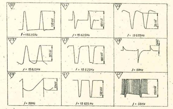
• MERANIE EL. VOLTMETROM JEJEDNOTNEHO HODNOTY NASTAVENI V ODBEROCH MF ZOSILNOVACA A VIDEOZOSILNOVACA SU MERANE BEZ SIGNALU P. NASTAVENI JASU A KONTRASTU NA MINIMU. OSTATNE HODNOTY NAPATI MERANE SO SIGNALOM PRI L 1 = 100% A KONTRASTU MAXIMALNY.
