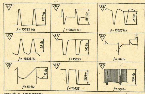
• MERANÉ EL. VOLTMETROM JEDNOHODNÉ HOODNOTY NAPÄTÍ V OBYCHODCH KANÁLOVÉHO VOLČIKA MF ZOSILŇOVAČA A VIDEOZOSILŇOVAČA SU MERANÉ BEZ SIGNÁLU PRI NASTAVENÍ JASU A KONTRASTU NA MINIMUM. OSTATNÉ HOODNOTY NAPÄTÍ MERANÉ SO SIGNÁLOM PRI I_{0} = 100 \mu A KONTRAST MAXIMALNY
