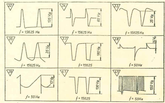
• MĚŘANÉ EL. VOLTMETROM • JEDNOMĚRNÉ HODNOTY NAPĚTÍ V OBVODOCH KANÁLOVÉHO VOLĚA MF ZOSILŇOVAČE A VIDEOZOSILŇOVAČA SÚ MĚŘANÉ BEZ SIGNÁLU. PRI NASTAVENÍ JASU A KONTRASTU NA MINIMUM. OSTATNÉ HODNOTY NAPĚTÍ MĚŘANÉ SO SIGNÁLOM PRI I_{KO} = 100 \mu A , KONTRAST MAXIMÁLNY.
