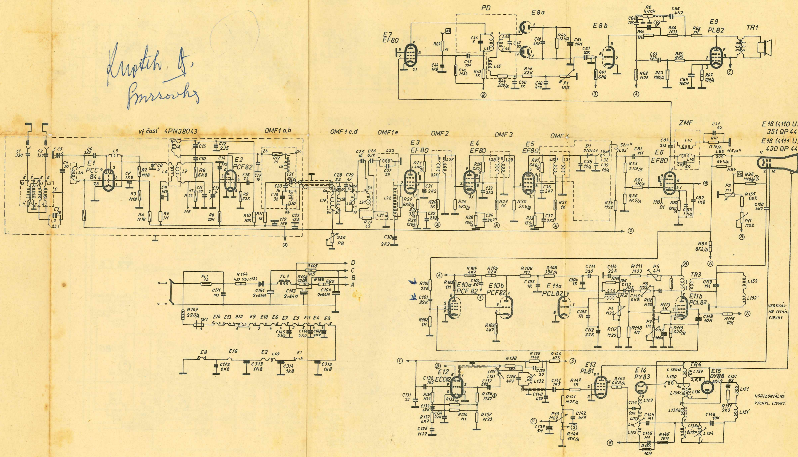
Obr. 7.16.* Schéma televizného prijímača Kravich 4111-U
