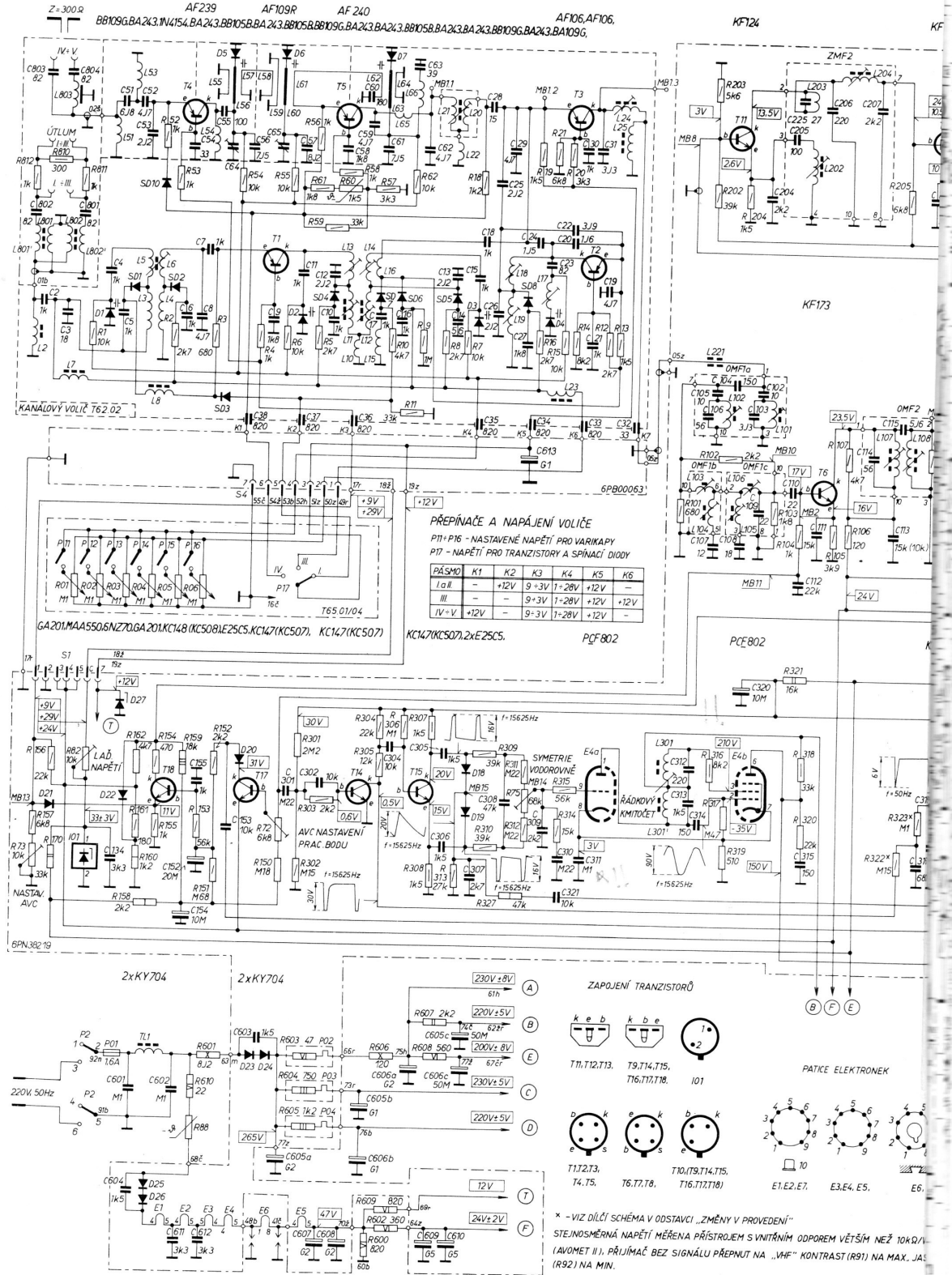
XVIII. Zapojení televizních přijímačů 4136U „CAVALLO“, 4249U „CASTELLO“ (poslední provedení) a 4256U „ZENIT“, 421
